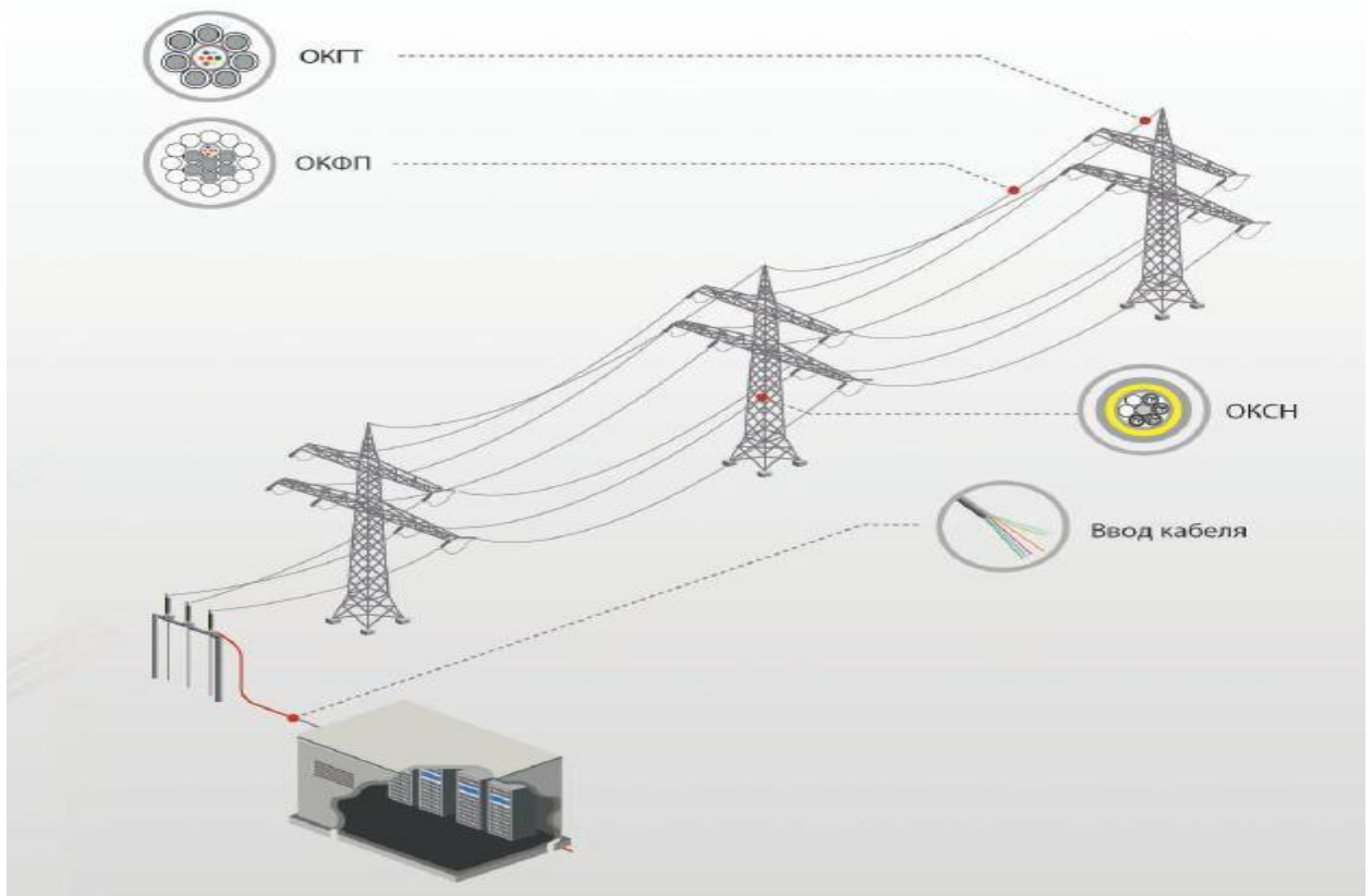
Рисунок 10. Пример использования самонесущего кабеля (ОКСН) и оптического кабеля, встроенного в фазный провод (ОКФП) и грозозащитный трос (ОКГТ)
